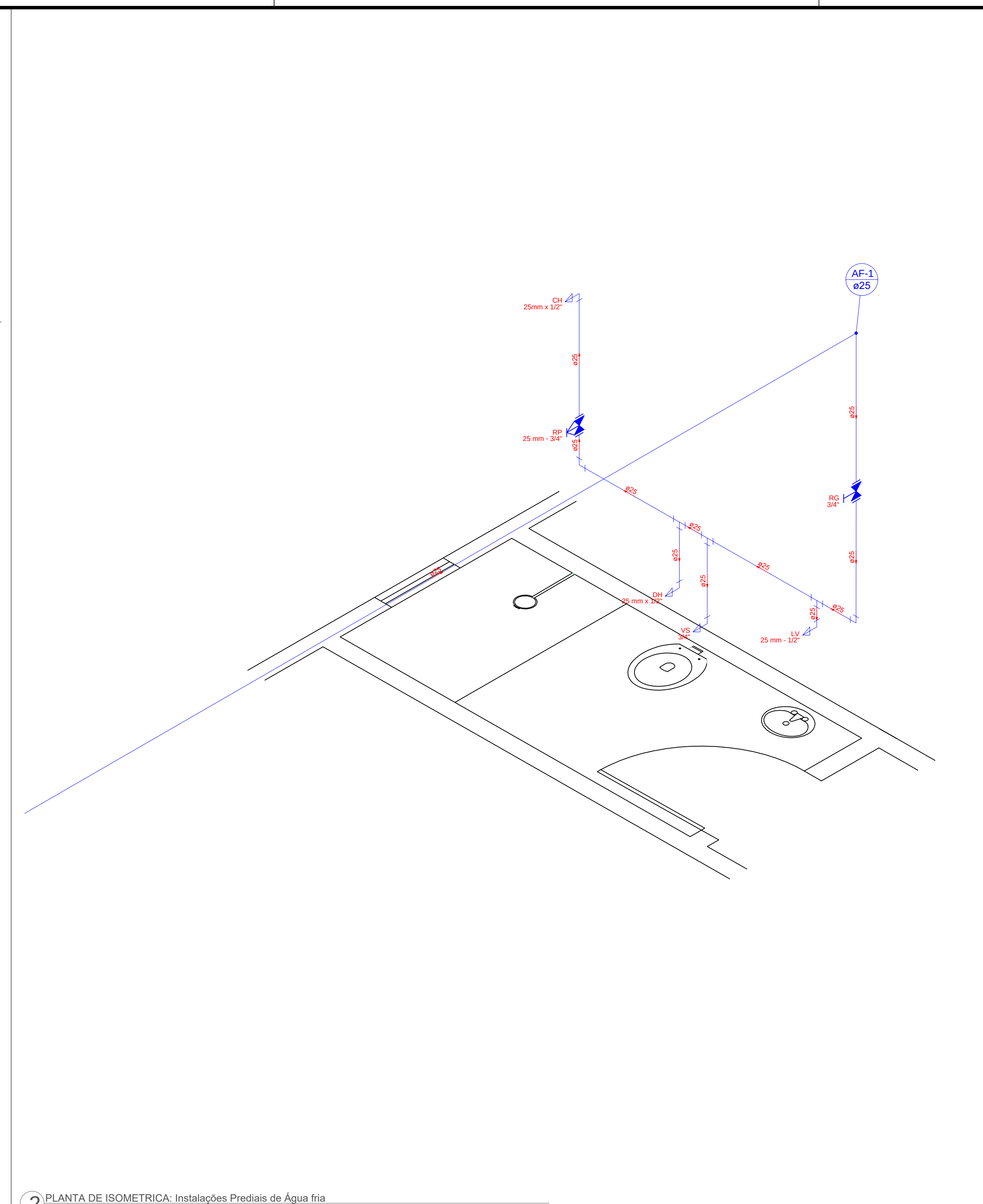
2 PLANTA DE ISOMETRICA: Instalações Prediais de Água fria
